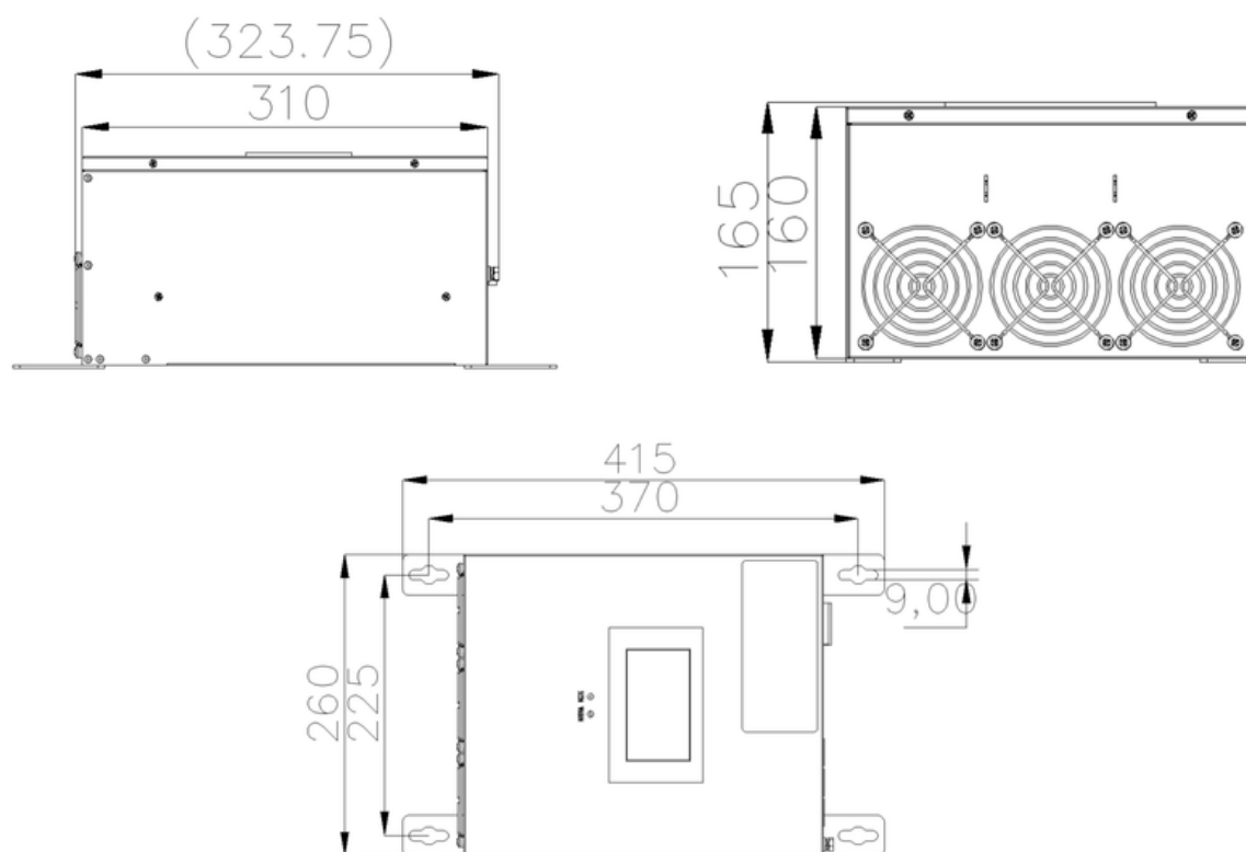
Rysunek 2. Wymiary kompensatora REACTO Mini mocy 5kVar.
